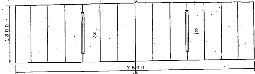
WEB FRAME SECTION
