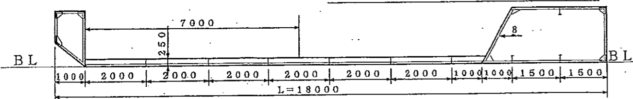
LONG FRAM SECTION
