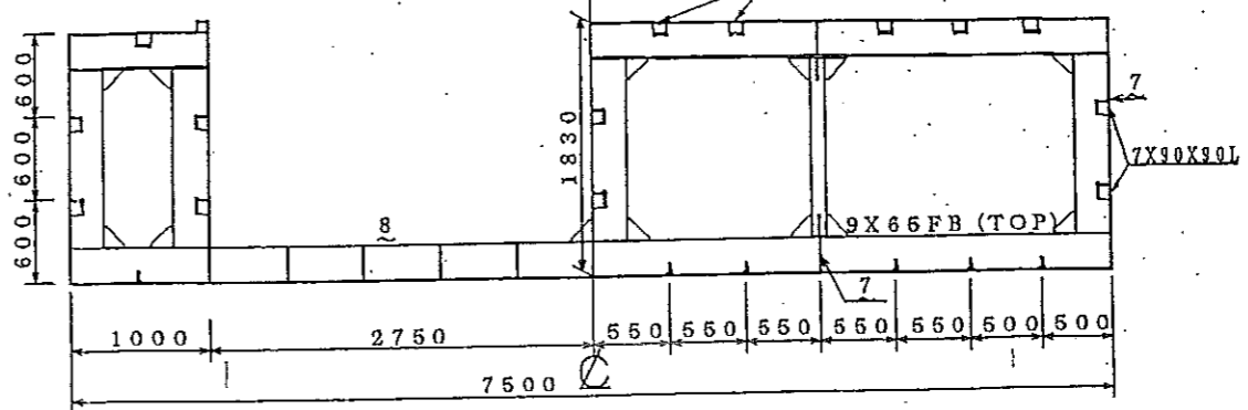
WEB FRAME SECTION
