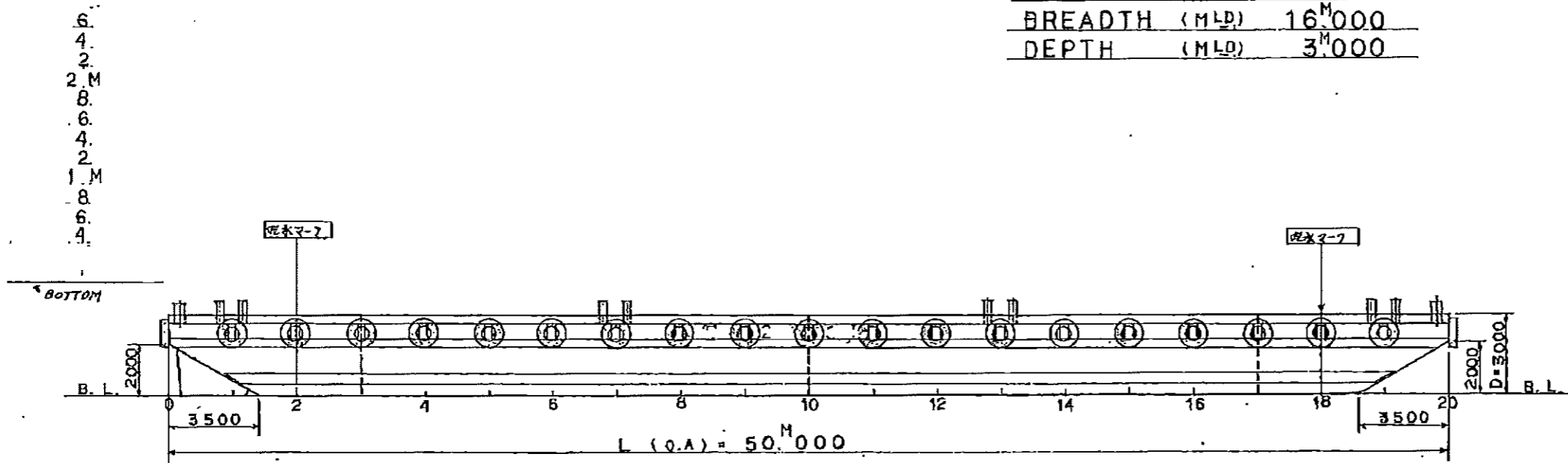
吃水マ-7 船首尾面図
