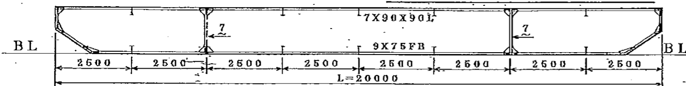
LONG FRAM SECTION
