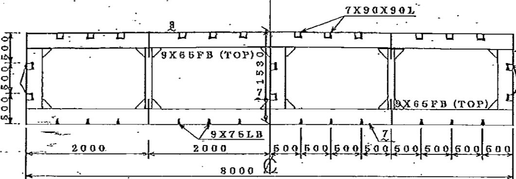
WEB FRAME SECTION
