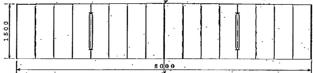
WEB FRAME SECTION
