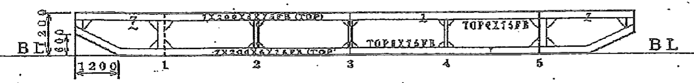
LONG FRAM SECTION
