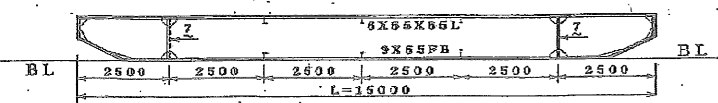
LONG FRAM SECTION
